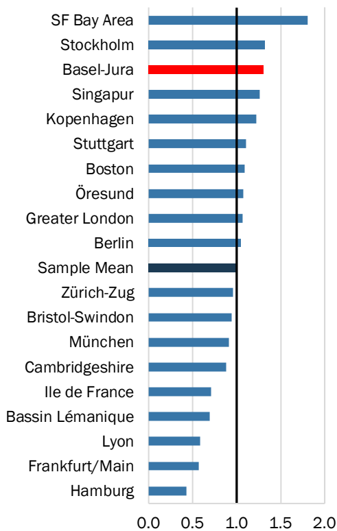
Abb. 1-13 Indexiertes BIP-Wachstum, 2013-2018
